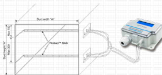
Abbildung 2. FloXact™ -L-Montage.
