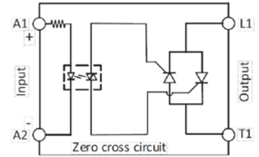
Anschlußplan:
